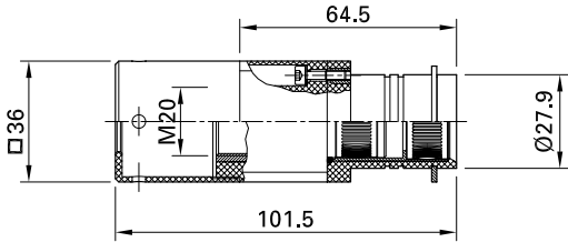
MGS1VB-M20-IS...
