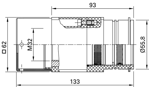
MGS3VB-M32-IS...
