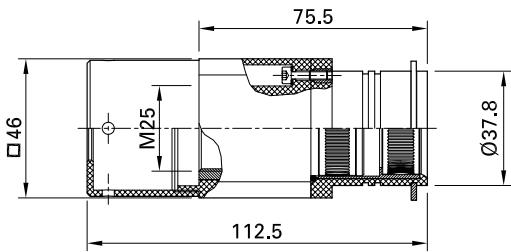
MGS2VB-M25-IS...
