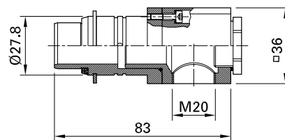
MGS1VS-M20
