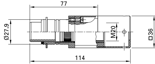
MGS1VS-M20-IS...
