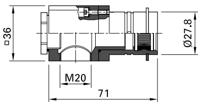
MGS1VB-M20
