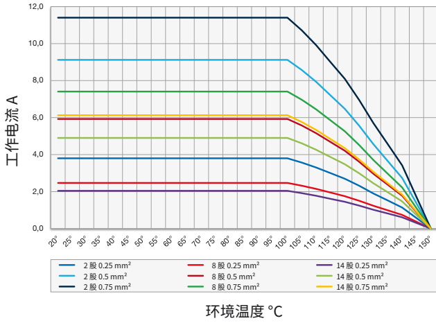
SIL: 电缆 0.25 mm 2 , 0.5 mm 2 & 0.75 mm 2
