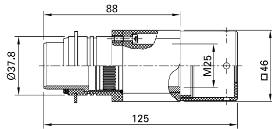
MGS2VS-M25-IS...
