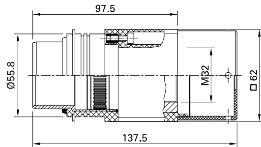
MGS3VS-M32-IS...
