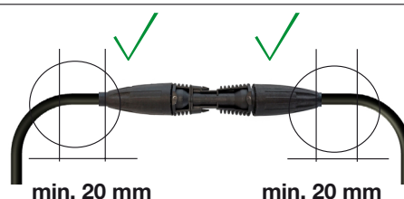
Correcte plaatsing van kabel Proper cable routing
