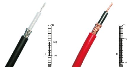
RG58-PVC
